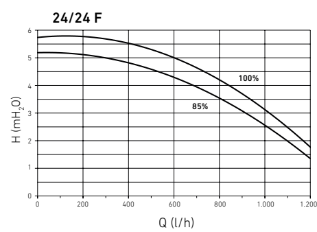
Presión disponible a la salida de la caldera.
