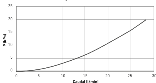
Pérdidas de carga de la unidad interior
